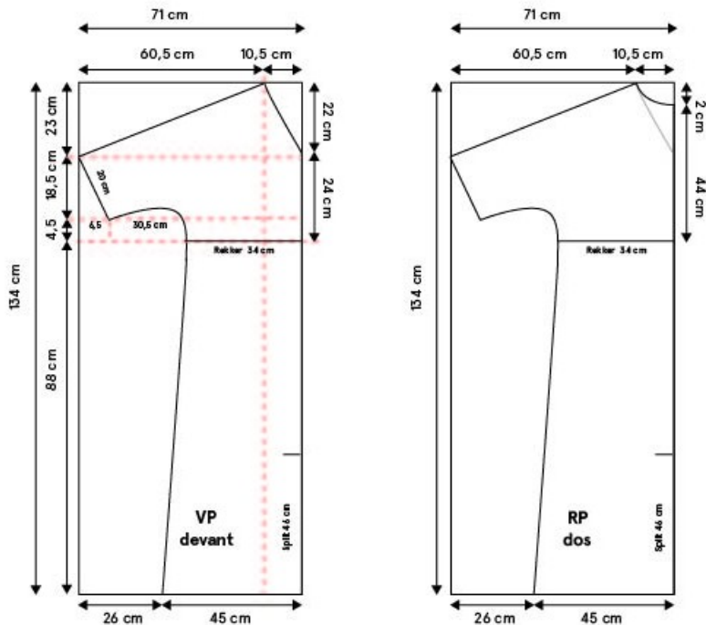
Poly - maxidress met mouw afmetingen patroon (in cm) dimensions patron (en cm)
