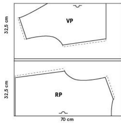
knipplan / plan de découpe
